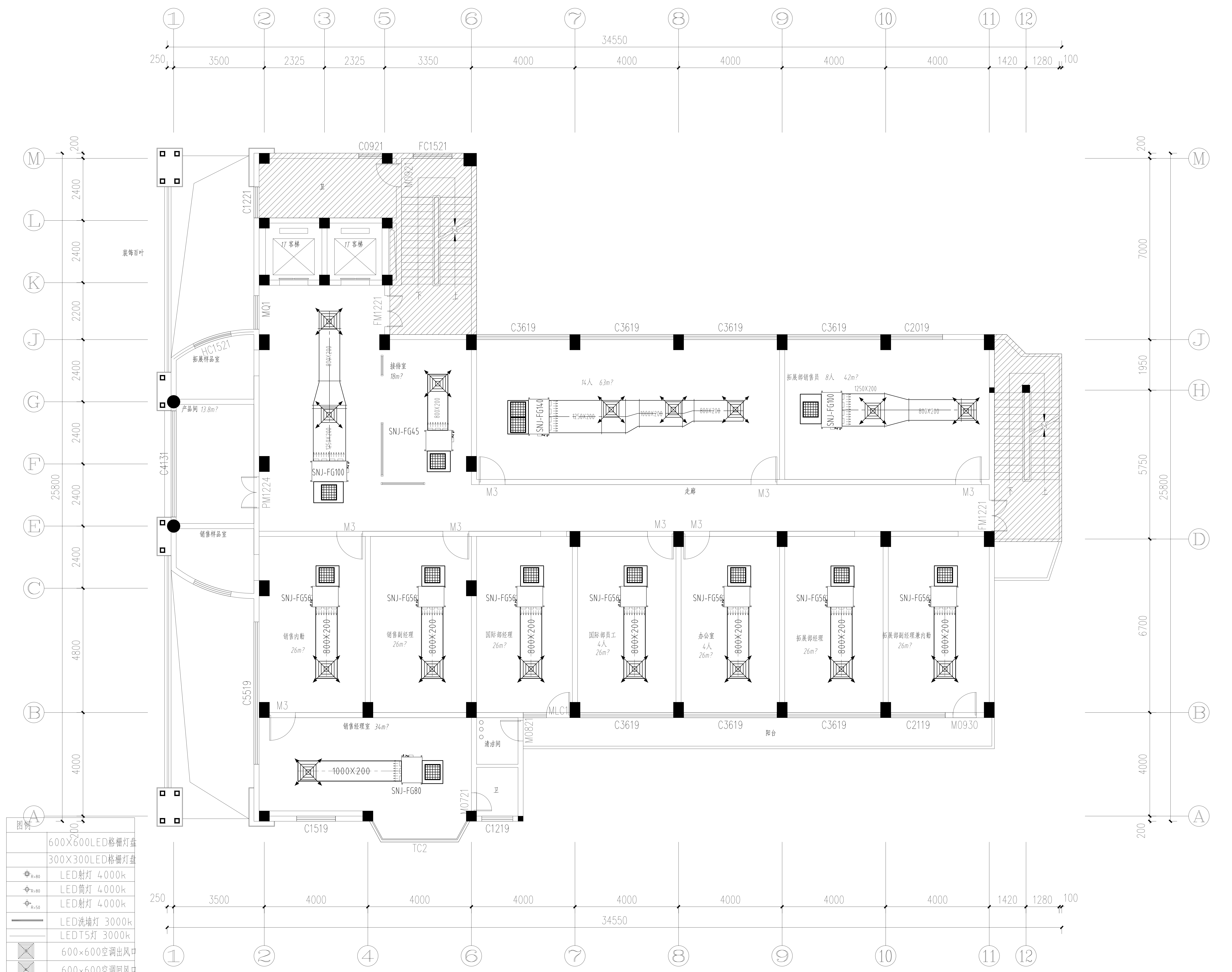
二层空调新风管道平面图 1:100
